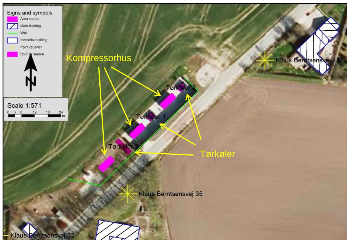
Figur 1 Layoutplan/oversigtskort for kompressor anlæg position nærliggende Klaus Berntsensvej, Særslev, Sønder sø.
